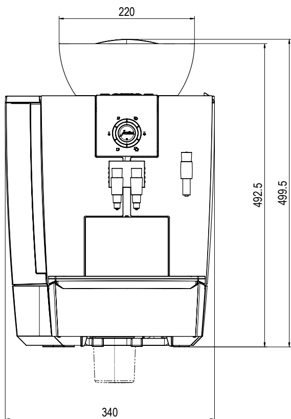
Vooraanzicht
