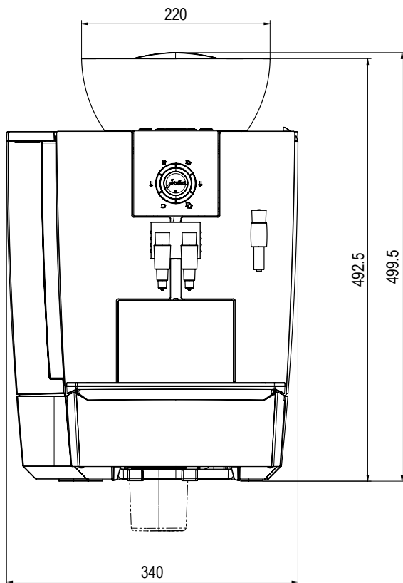
Aufriss
