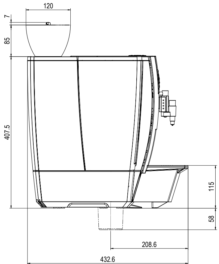
Seitenriss
