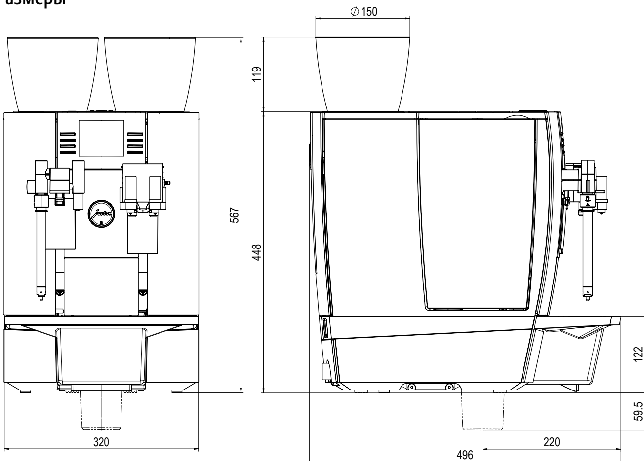
Вид спереди
