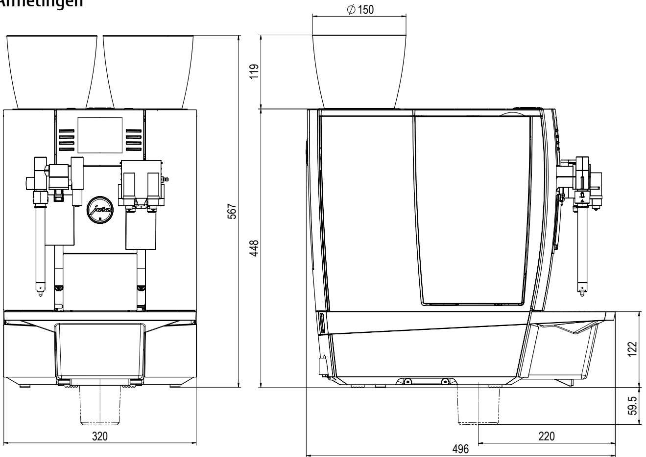
Vooraanzicht
