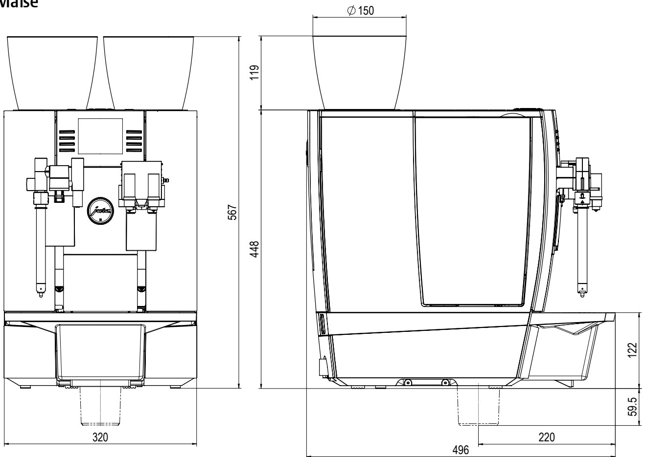
Aufriss
