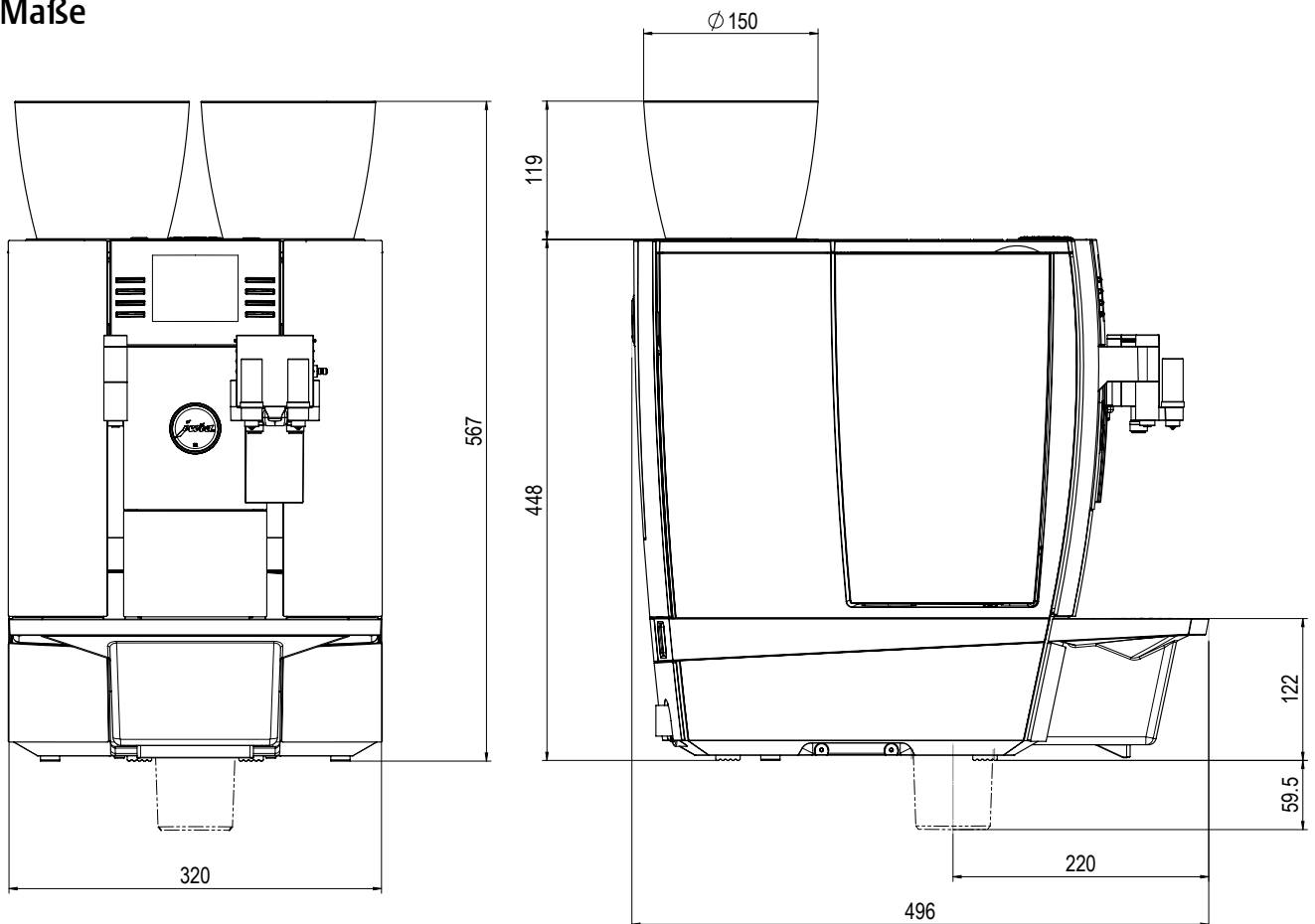
Aufriss
